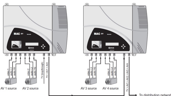
zapojení dvou modulátorů MAC-201 do kaskády
