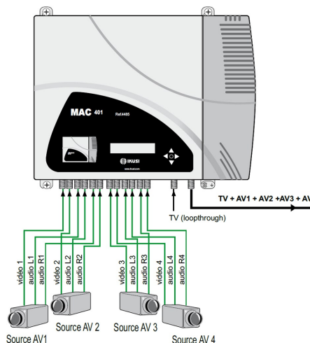
zapojení MAC-401
